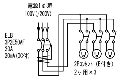
結線図
